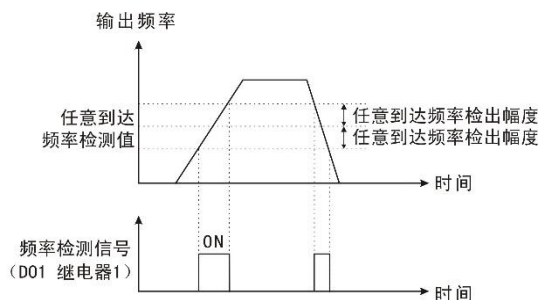
图 8-8-5 任意到达频率检测示意图
