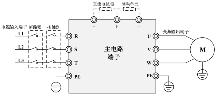
图 4-2-1 主电路端子示意图
