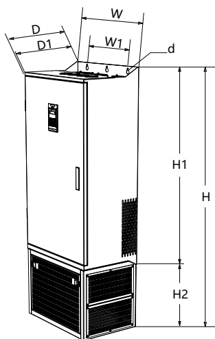
图 4-1-2 外形尺寸
