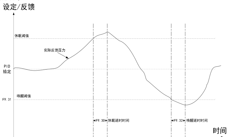
图 8-9-2 PID 休眠与唤醒时序示意图
