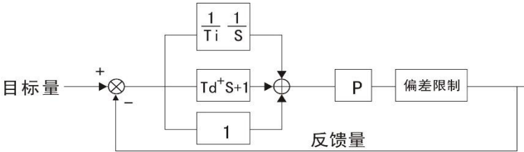
图 8-9-1 过程 PID 原理框图
