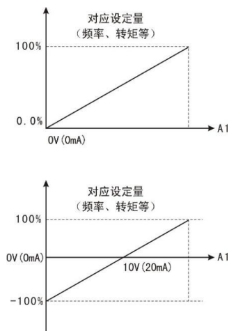
图 8-5-1 模拟给定与设定量的对应关系
