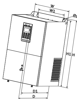
图 4-1-1 外形尺寸
