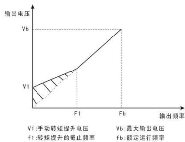
图 8-4-1 手动转矩提升示意图
