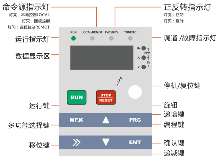
图 2-1-1 操作面板示意图
