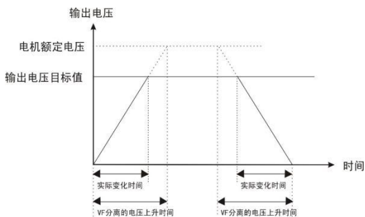
图 8-4-3 V/F 分离示意图
