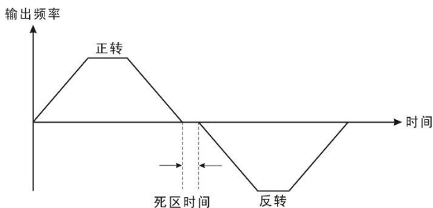
图 8-8-2 正反转死区时间示意图
