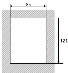
图 3-1-2 面板开孔尺寸示意图
