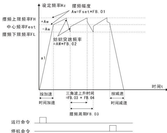
图 8-B-1 摆频工作示意图
