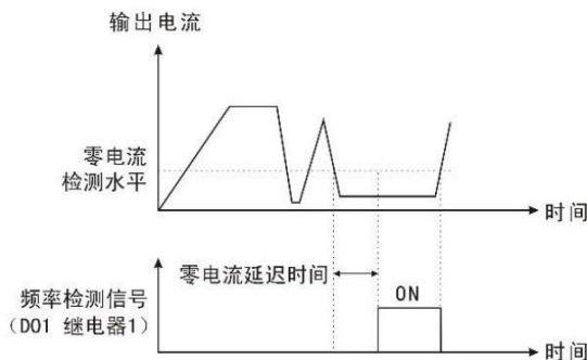
图 8-8-7 零电流检测示意图
