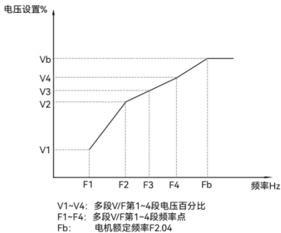
图 8-4-2 V/F 曲线设定示意图
