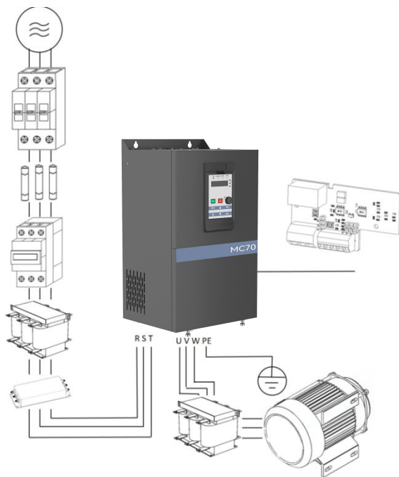
图 1-5-1 系统构成图
