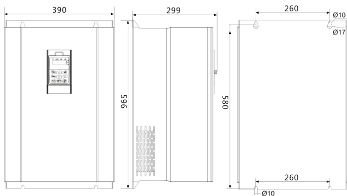
75kW ~ 110kW 外型尺寸及安装尺寸示意图
