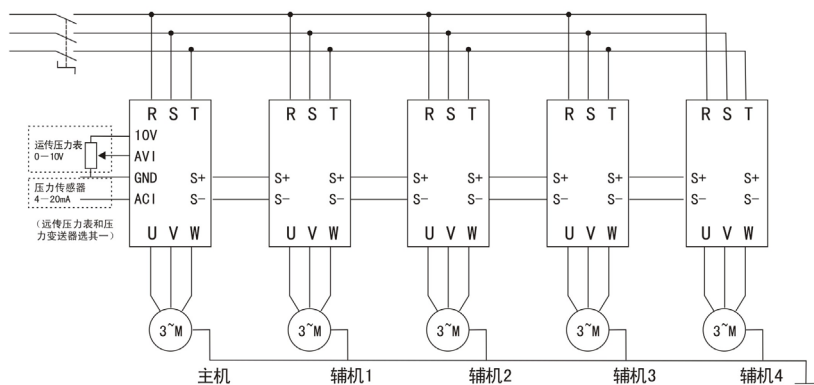
端子接线图
