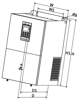
图 2-3-2 外形尺寸 2
