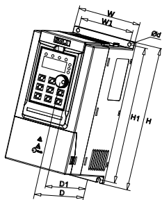
图 2-3-1 外形尺寸 1
