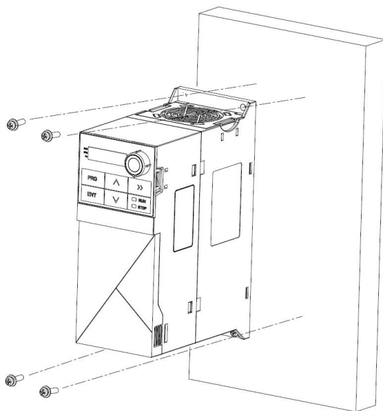
图 5-2-1 螺钉安装示意图
