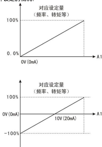
图 9-5-1 模拟给定与设定量的对应关系
