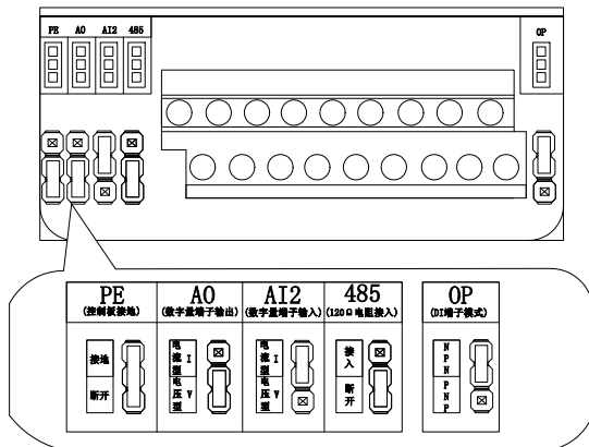
图 4-5-3 跳线端子功能示意图 2
