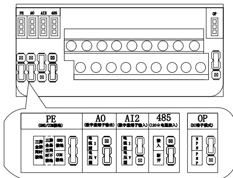
图 4-5-2 跳线端子功能示意图 1
