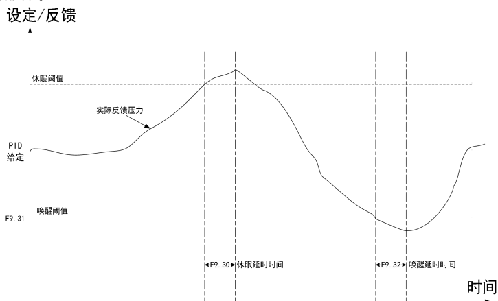
图 9-9-2 PID 休眠与唤醒时序示意图
