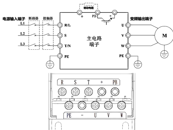
图 4-4-1 主电路端子示意图
