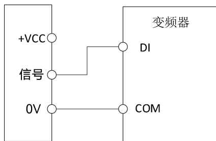
图 5-4-3 DI 漏型（NPN）供电接线示意图
