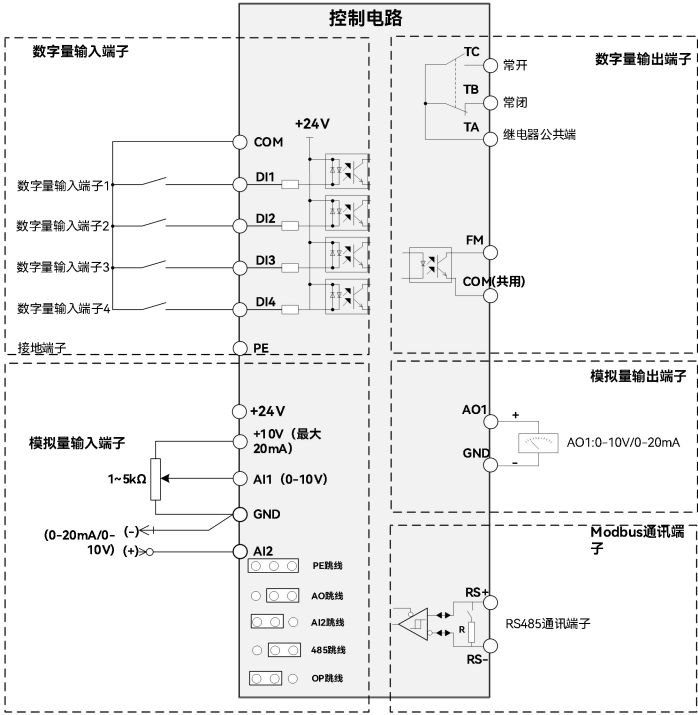
图 4-5-1 控制回路端子示意图
