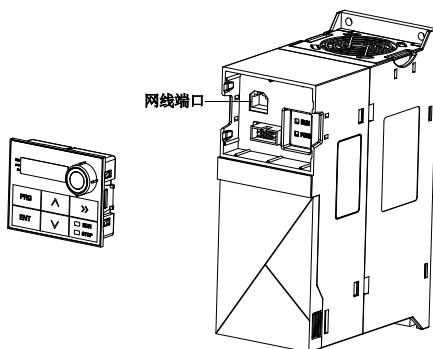
图 3-1-3 外引键盘示意图
