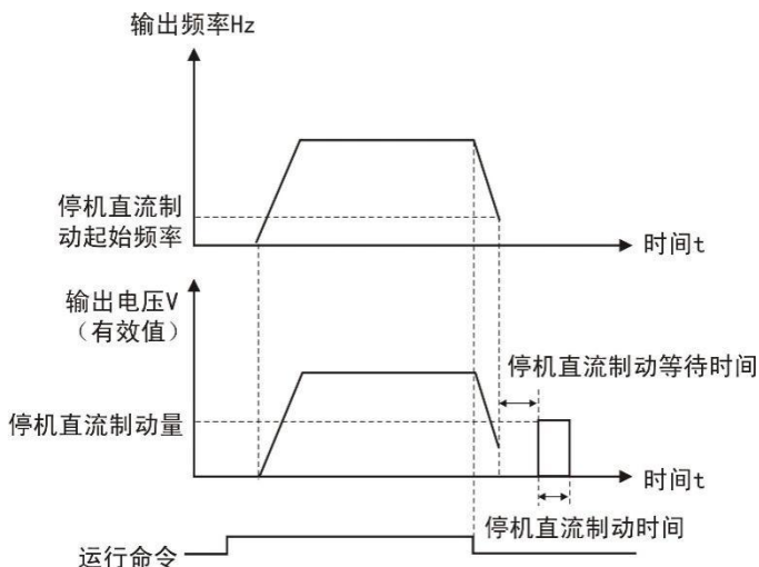
图 9-1-1 停机直流制动示意图
