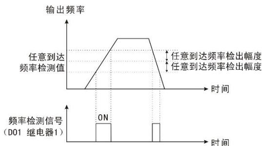
图 9-8-5 任意到达频率检测示意图
