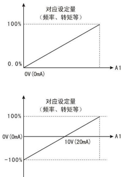
图 9-5-1 模拟给定与设定量的对应关系
