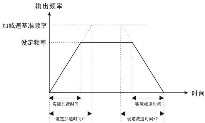
图 9-0-1 加减速时间示意图
