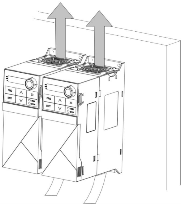
图 5-1-2 多台机器并排安装
