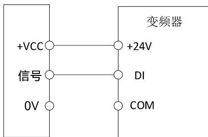
图 5-4-3 DI 漏型（NPN）供电接线示意图
