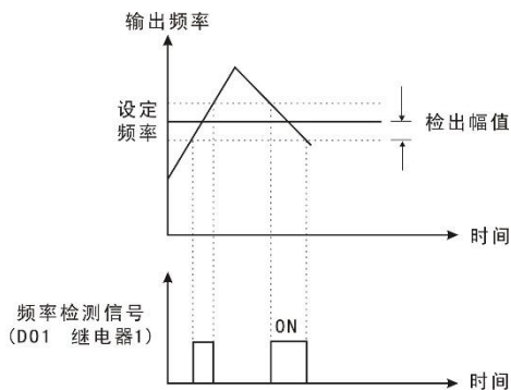
图 9-8-4 频率到达检出幅值示意图
