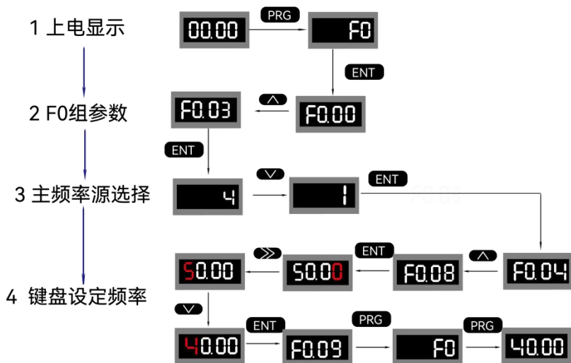
图 2-2-1 快速调试流程
