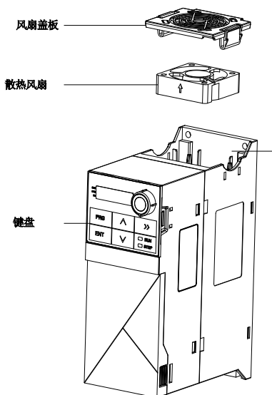
图 3-1-5 独立风扇可拆卸示意图
