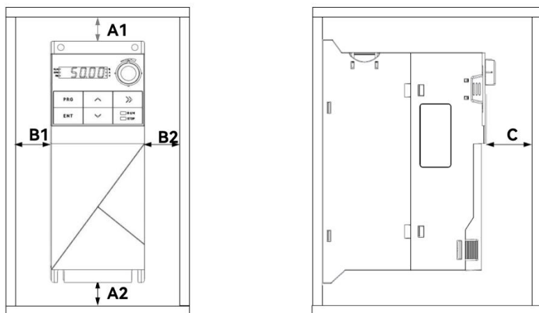
单台机器安装空间
