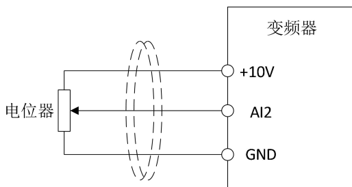
图 5-4-1 电压型接线示意图
