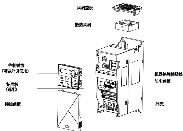
图 3-1-1 产品部件示意图
