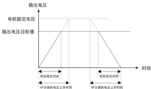
图 9-4-3 V/F 分离示意图
