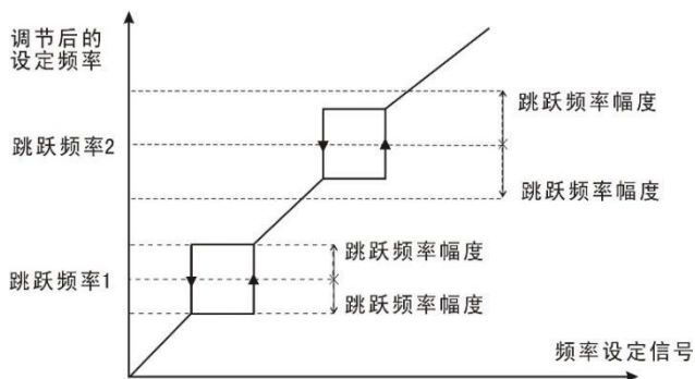
图 9-8-1 跳跃频率示意图
