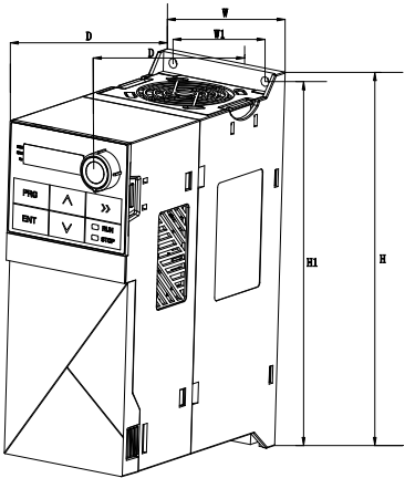
图 4-1-1 外形尺寸 V1
