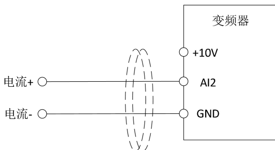
图 5-4-2 电流型接线示意图
