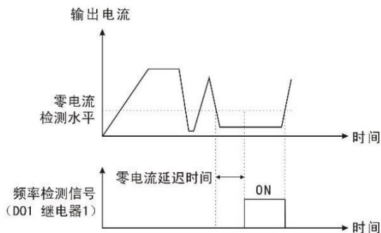
图 9-8-7 零电流检测示意图
