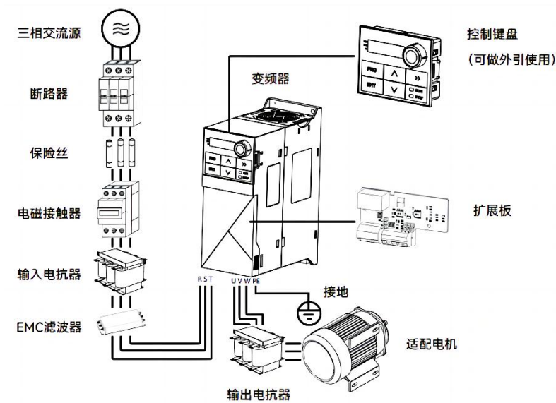
图 1-5-1 系统构成图
