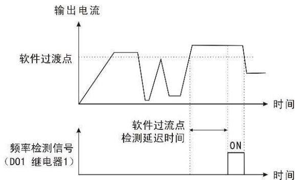
图 9-8-8 软件过流点检测示意图
