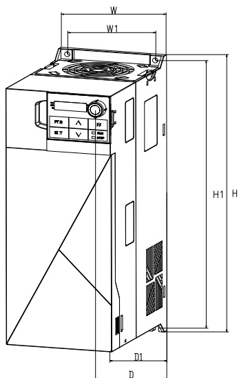
图 4-2-3 外形尺寸
