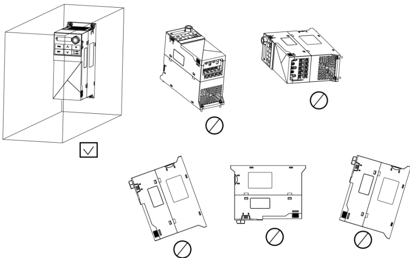
图 5-1-4 安装方向示意图
