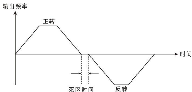
图 9-8-2 正反转死区时间示意图
