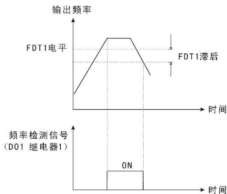
图 9-8-3 FDT1 电平示意图
