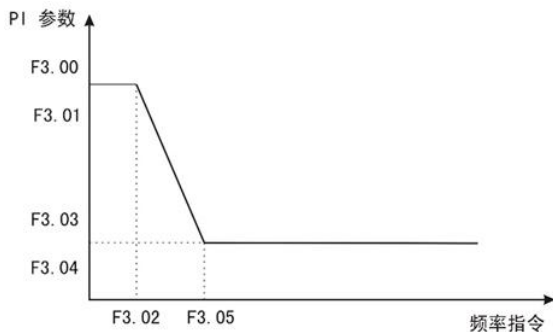
图 9-3-1 PI 参数示意图
