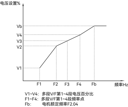
图 9-4-2 V/F 曲线设定示意图
