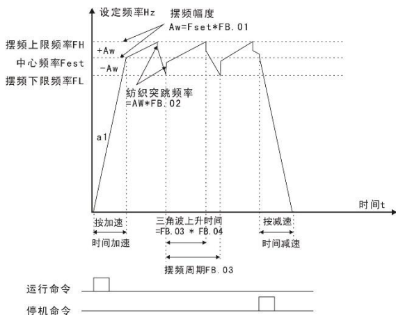
图 9-B-1 摆频工作示意图
