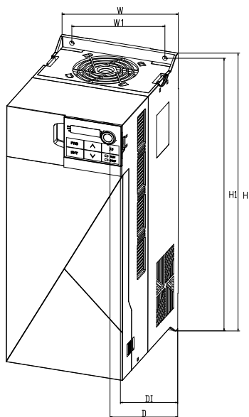
图 4-2-5 外形尺寸
