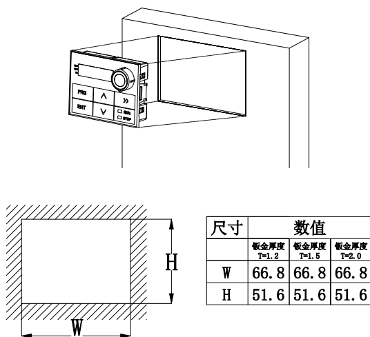
图 3-1-2 面板开孔尺寸示意图
