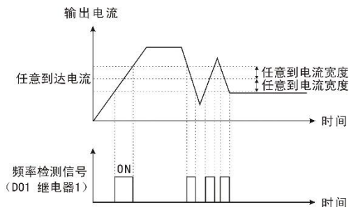
图 9-8-6 任意到达频率检测示意图
