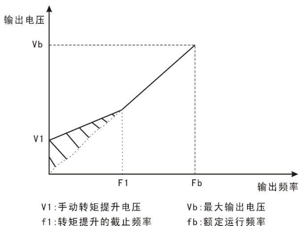
图 9-4-1 手动转矩提升示意图
