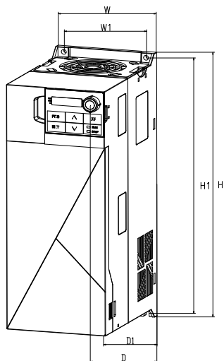
图 4-2-2 外形尺寸
