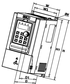
图 2-1-1 外形尺寸 1
