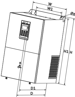
图 2-2-2 外形尺寸 2
